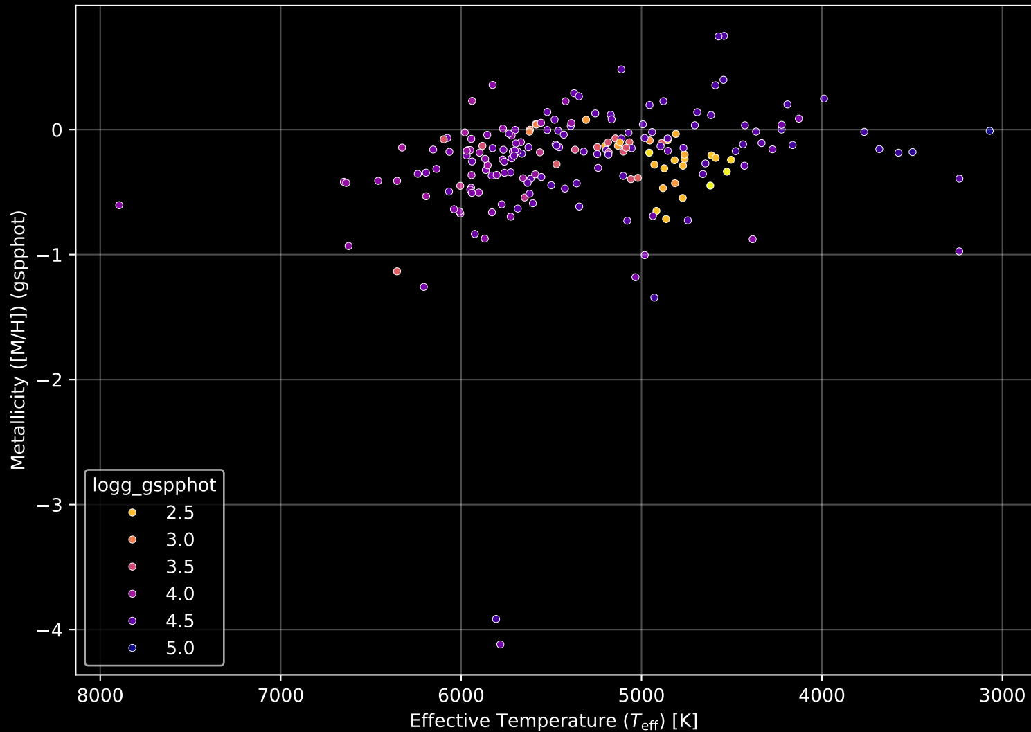
APOGEE DR17 Field: [143+76_MGA] Stellar Population Parameters (n= 197)
